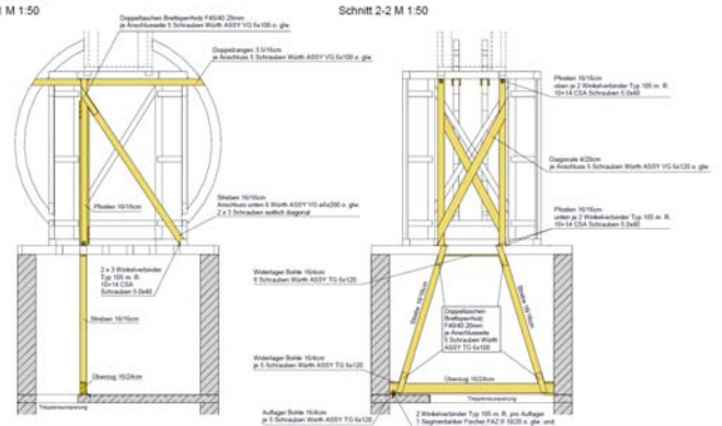
Stützkonstruktion Schnitt 1-1 M 1:50
